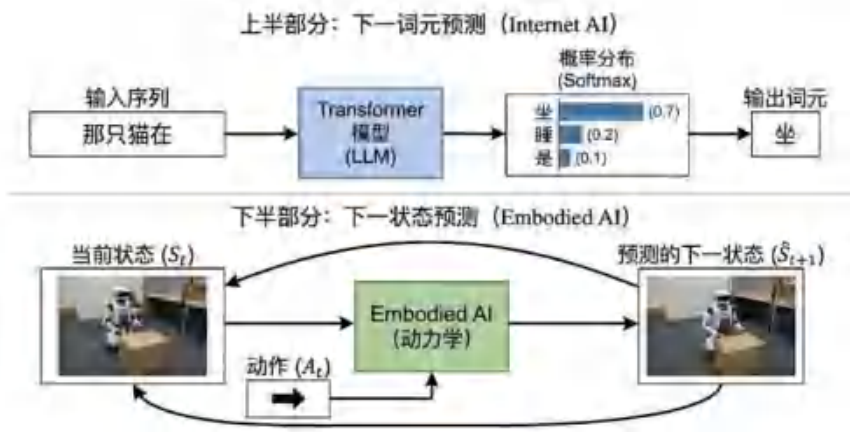
图 2.2: 下一词元预测与下一状态预测范式的对比
