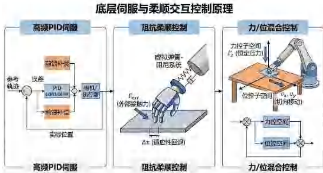
图 2.14: 底层伺服与柔顺交互控制原理
