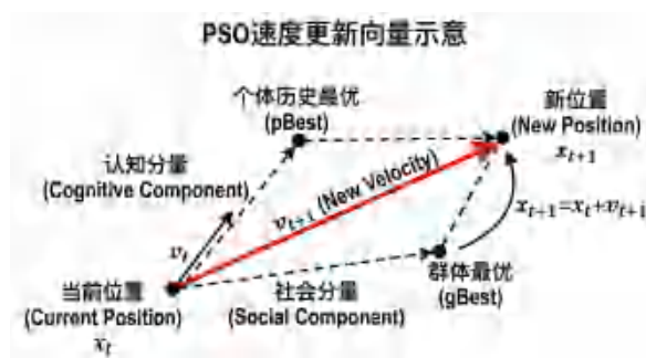
图 2.10: PSO 原理图
