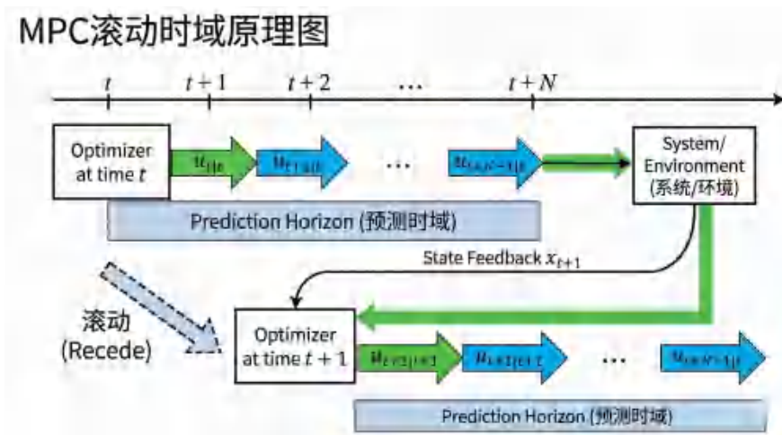
图 2.7: 滚动时域优化与 MPC 闭环控制原理
